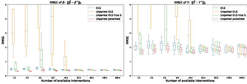
(a) RMSE: left \|\hat{\beta} - \beta^*\|_2 , right \|\hat{Y} - Y^*\|_2
